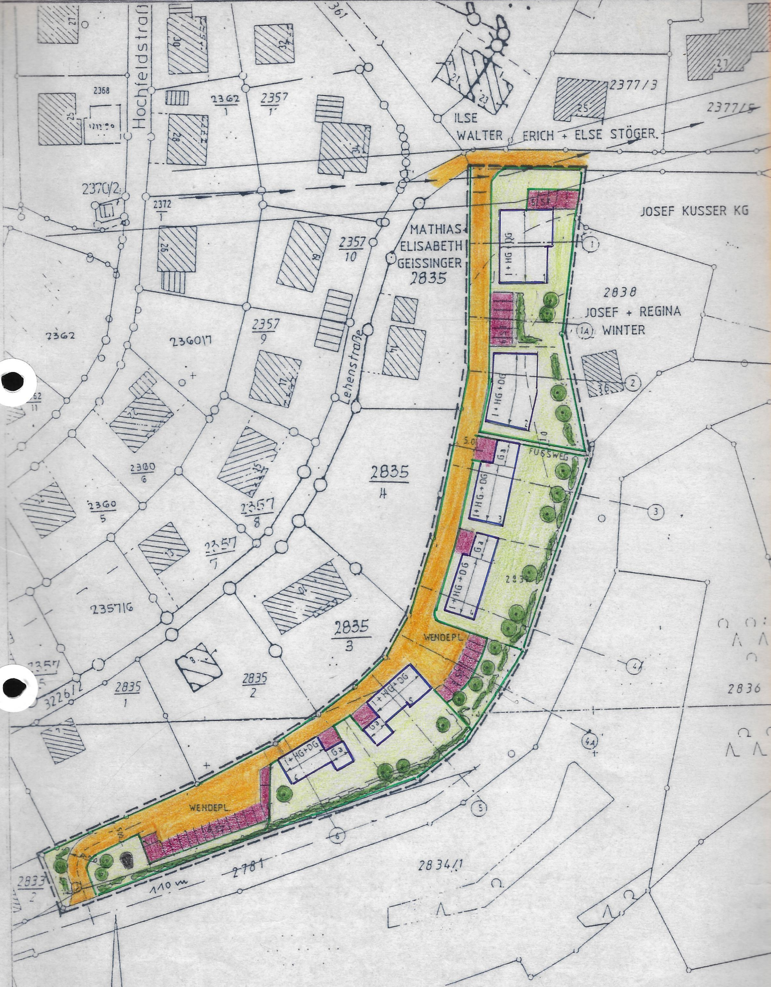
BEBAUUNGSPLAN NAMMERING M 1:1000
