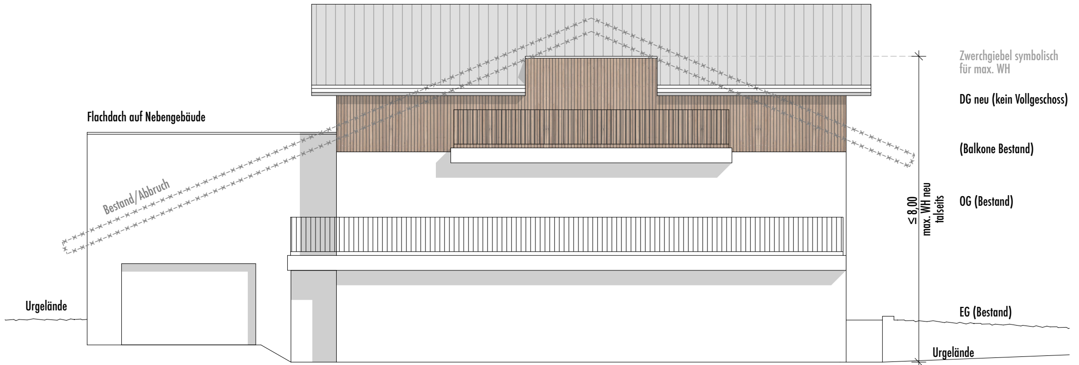
SCHEMAANSICHT SÜD
