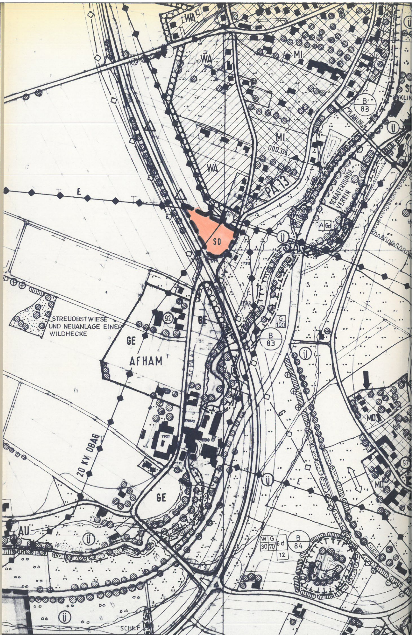
ÜBERSICHTSLAGEPLAN
