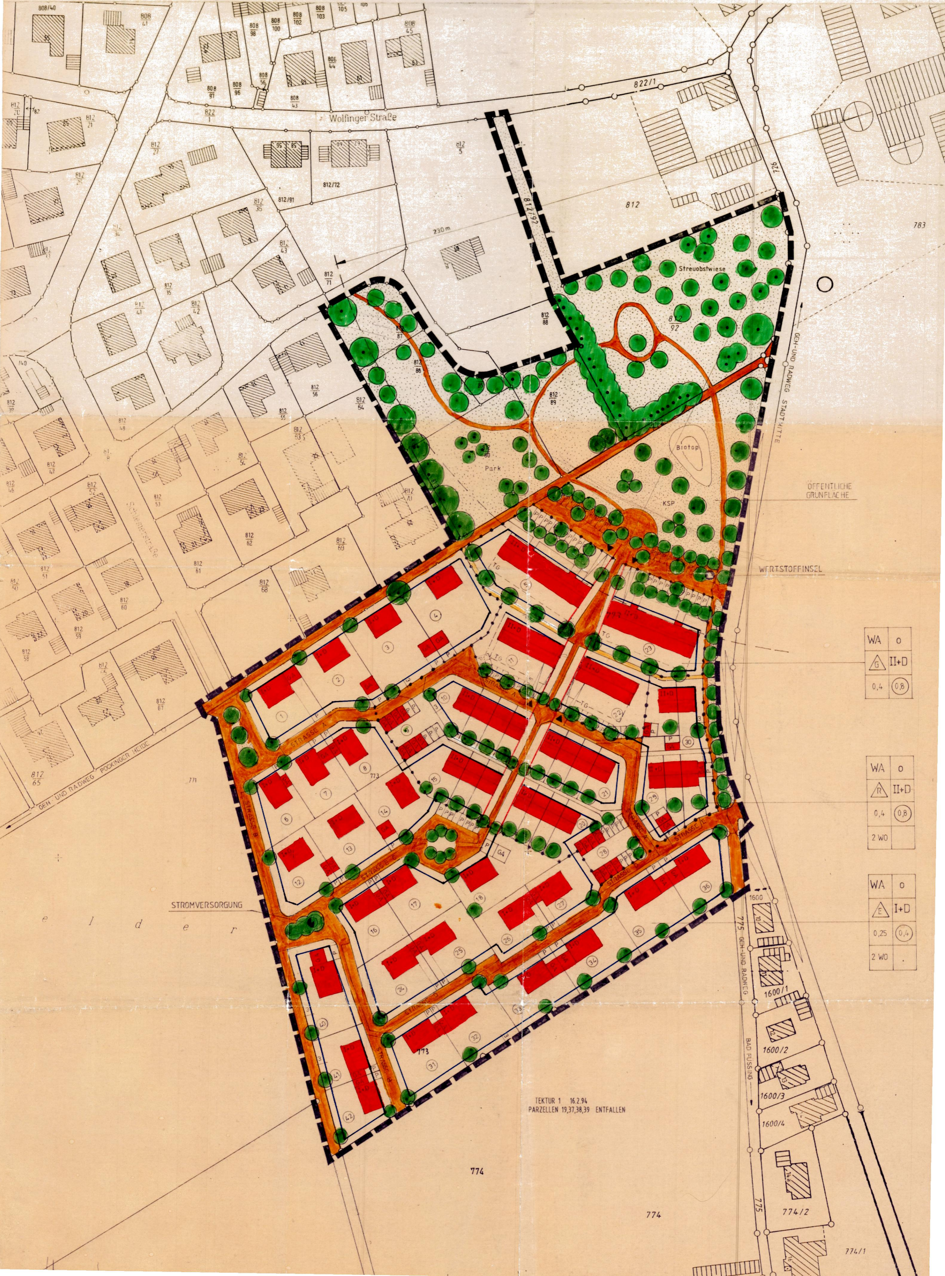
BEBAUUNGSPLAN 1/1000
