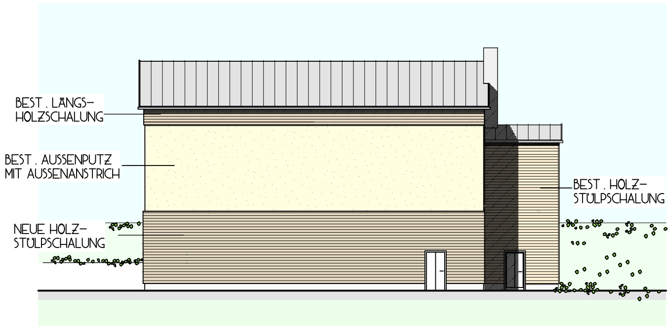
ANSICHT VON WESTEN M 1:200
