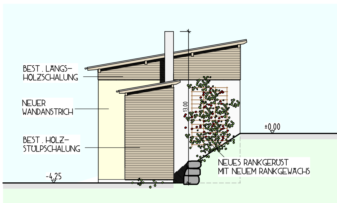
ANSICHT VON SÜDEN M 1:200
