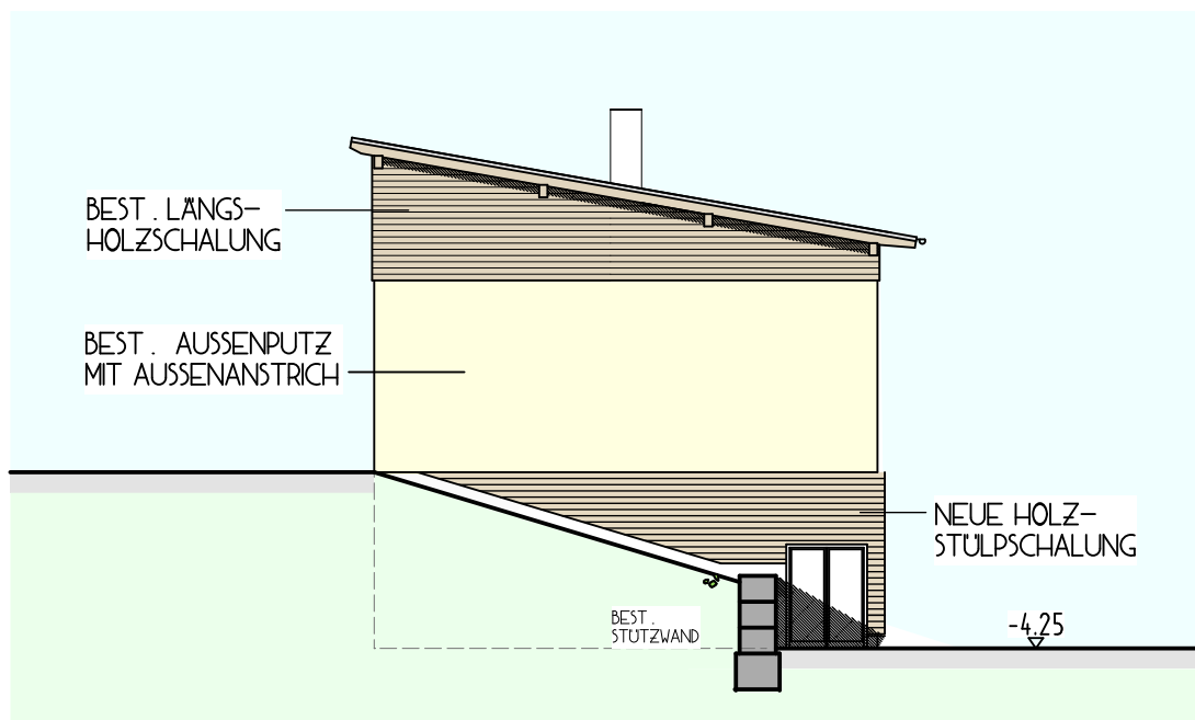
ANSICHT VON NORDEN M 1:200
