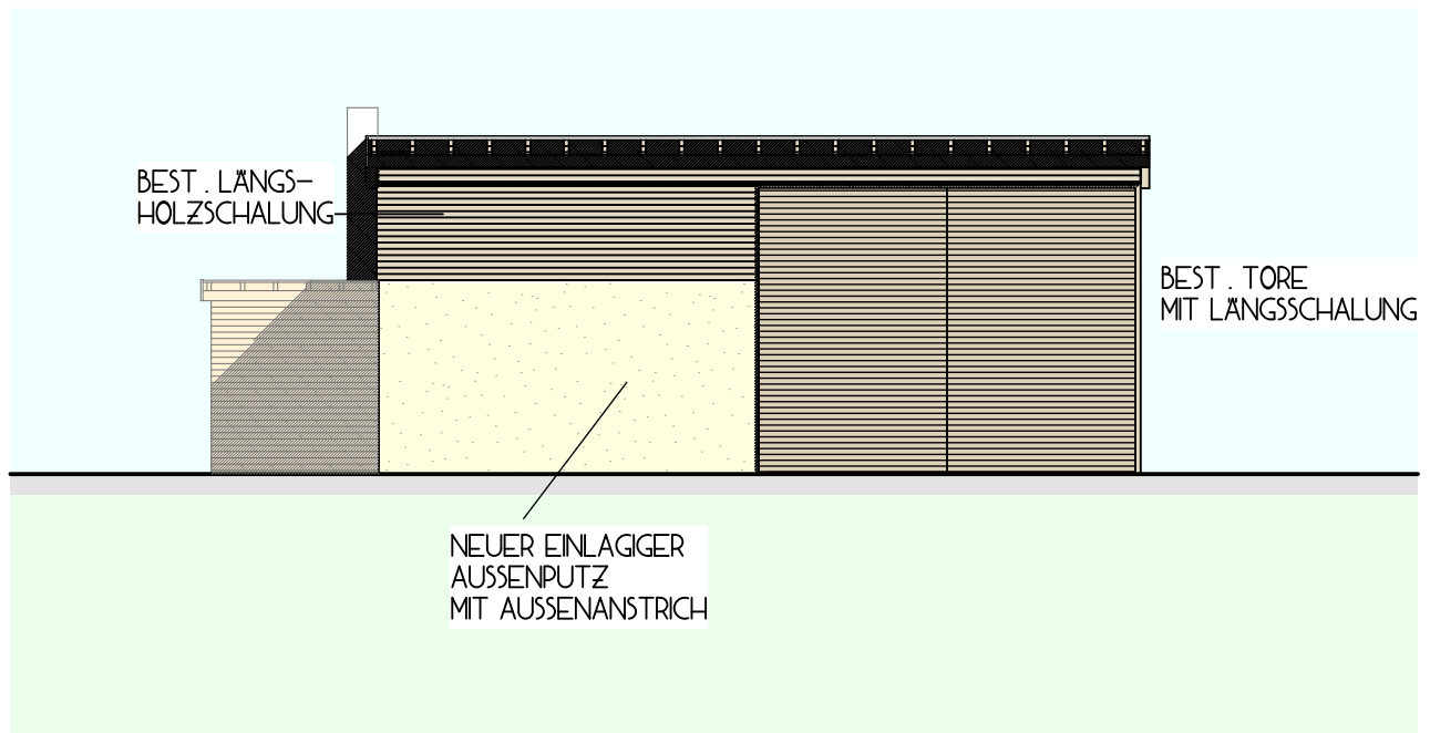
ANSICHT VON OSTEN M 1:200
